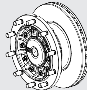
B-Serie (AirVent-Radkopf) mit Scheibenbremsen für Räder Single ET120
