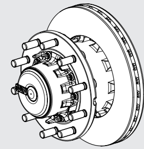
S- und Z-Serie mit Scheibenbremsen für Räder Single ETO/Zwilling
