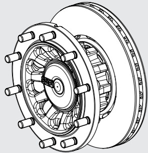
BI-Serie (INTEGRAL-Radkopf) mit Scheibenbremsen für Räder Single ET120
